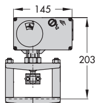
Actuator E1 Types 5824 and 5825
